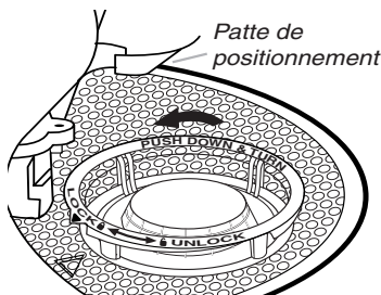
Dépose du filtre supérieur
